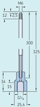
Verlängerungsrohr mit M6-Gewinde
