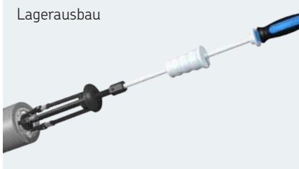
Lagerausbau
